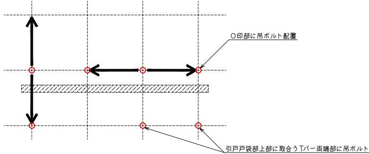
グリッドTバーから外れた位置に取り合う場合の振れ止補強（例）
