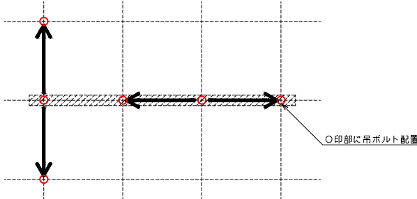
グリッドTバー直下に取り合う場合の振れ止補強（例）
