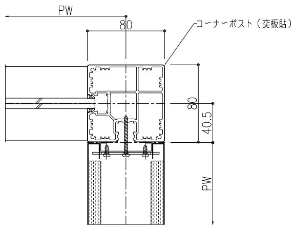
コーナーポスト
