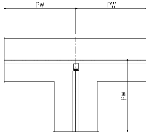
連装ガラス3WAY
