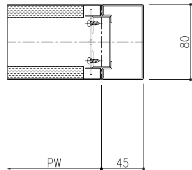
フリーエンド (パネル)
