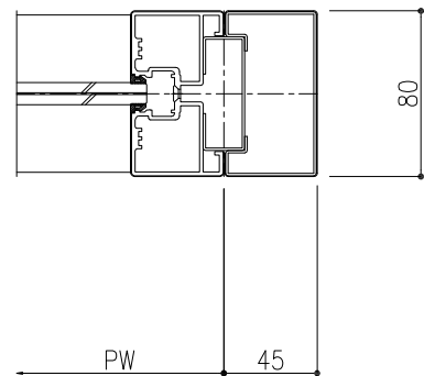
フリーエンド (ガラスパネル)
