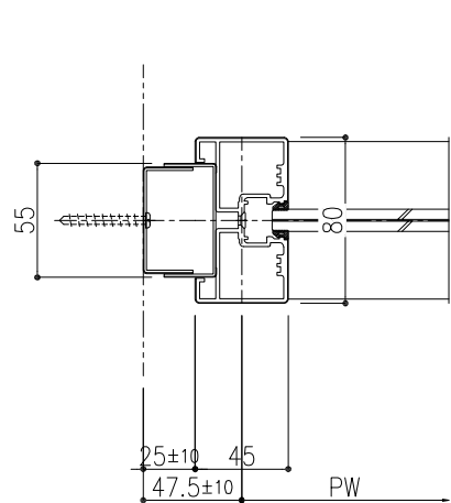
壁面取り合い (ガラス)
