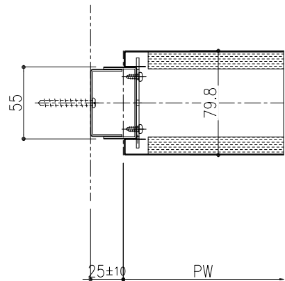
壁面取り合い (ガラス)
