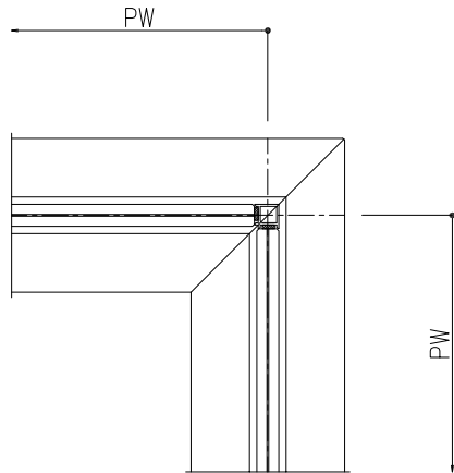
連装ガラスコーナー
