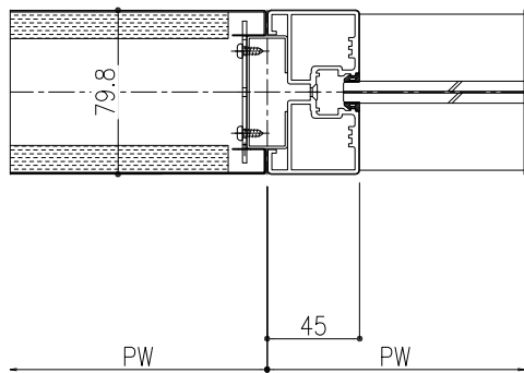
直線取り合い (パネル×ガラス)
