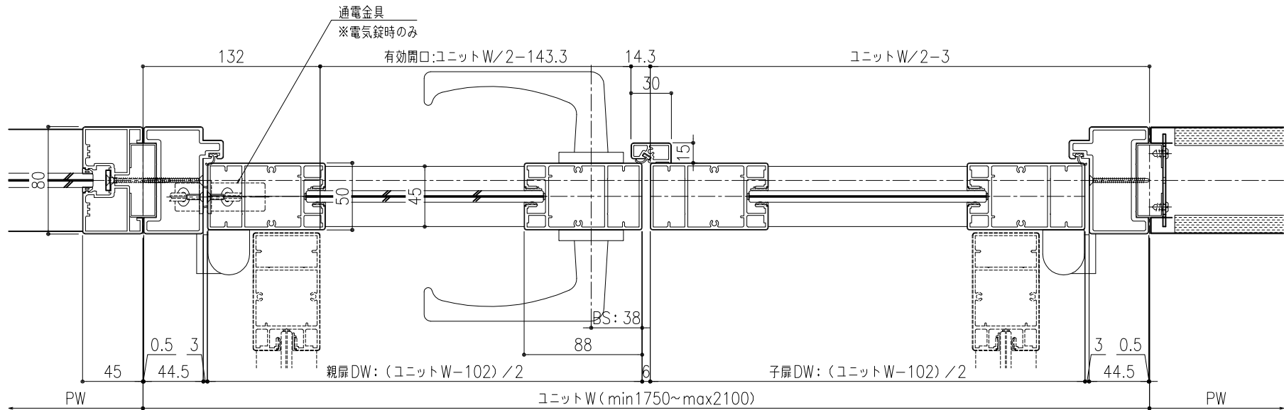
①-① ドアパネル平面断面図
