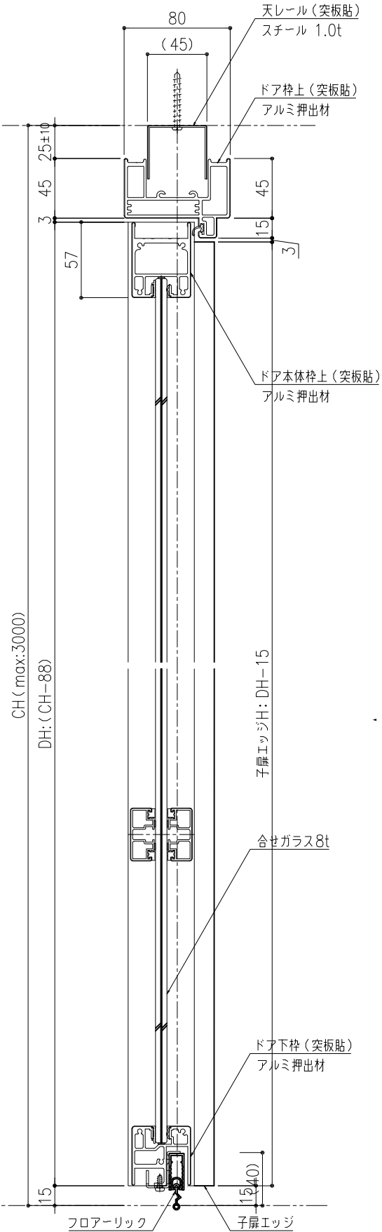
③-③ 断面図 (子扉)
