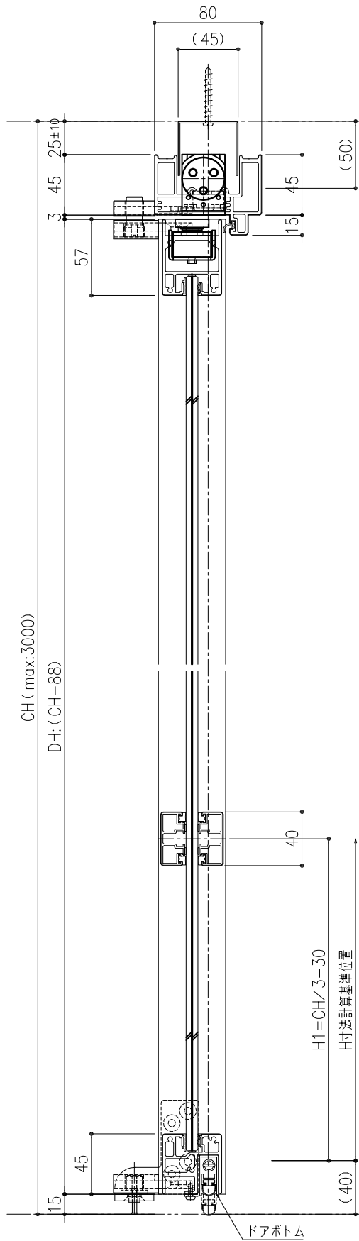
②-② 断面図 (親扉)
